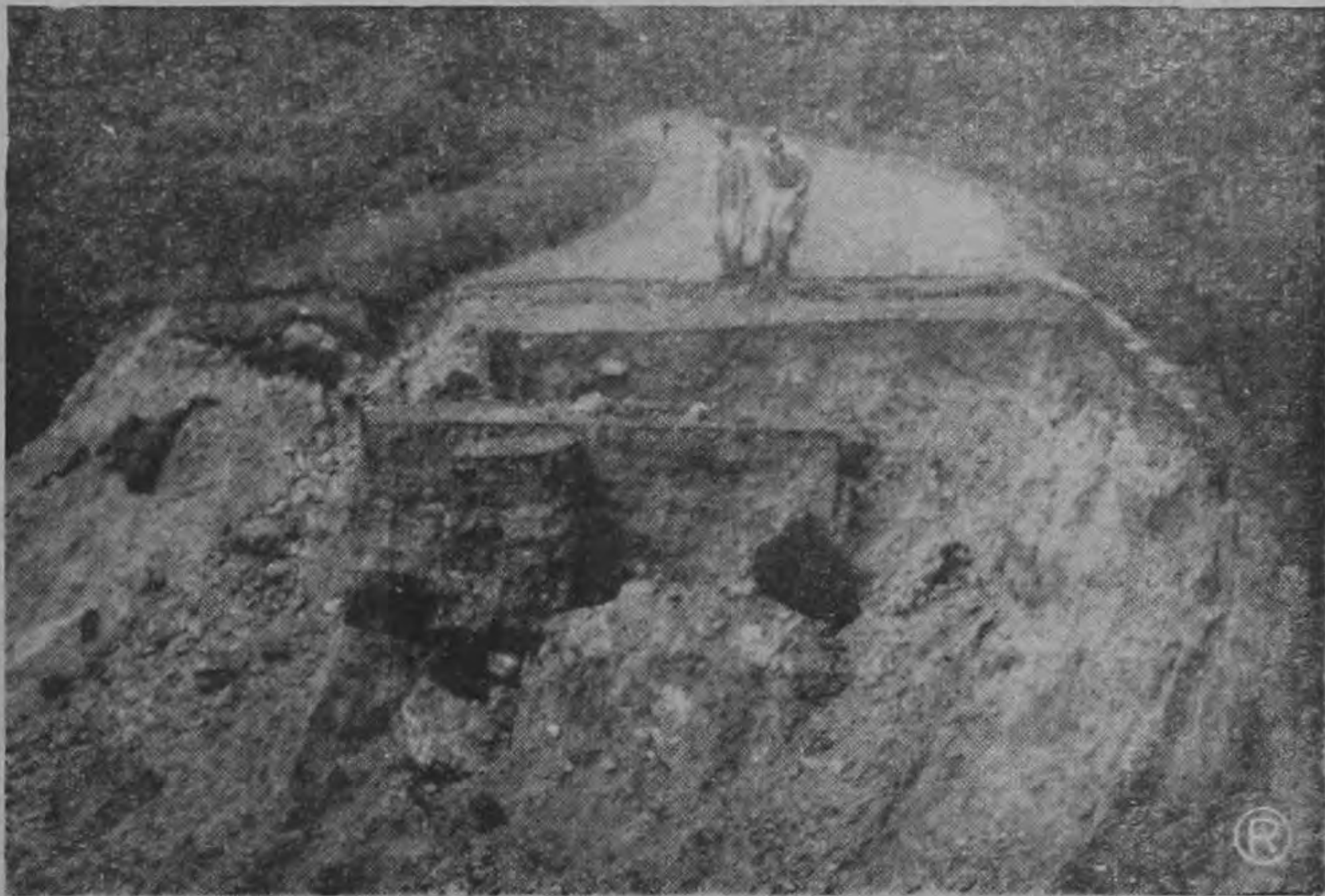
HUNDIMIENTO EN LA CARRETERA INTERAMERICANA.— Los Ingenieros Carlos Espinach y Fernando Sánchez observan el hundimiento en la Carretera Interamericana, ocurrido recientemente debido a los fuertes temporales. Véase la carretera trunca, quedando un abismo en el lugar donde antes pasaba la vía internacional. Obras Públicas estudia el terreno para realizar las reparaciones a la mayor brevedad posible. (Foto Tristán)
